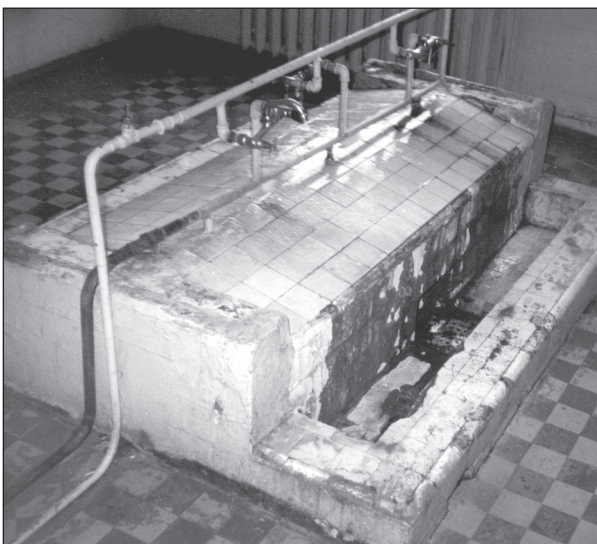
Primitieve toestanden.
