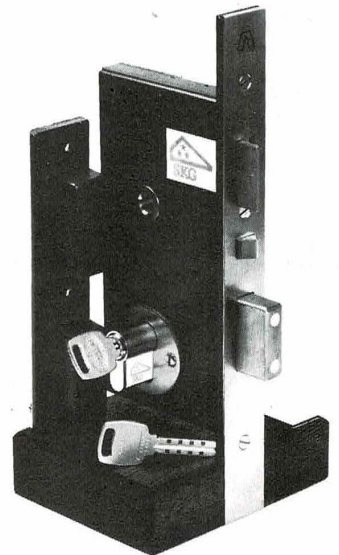
Extra zwaar cilinder-insteekslot met dag- en nachtschoot en bijbehorende sluitkom.
