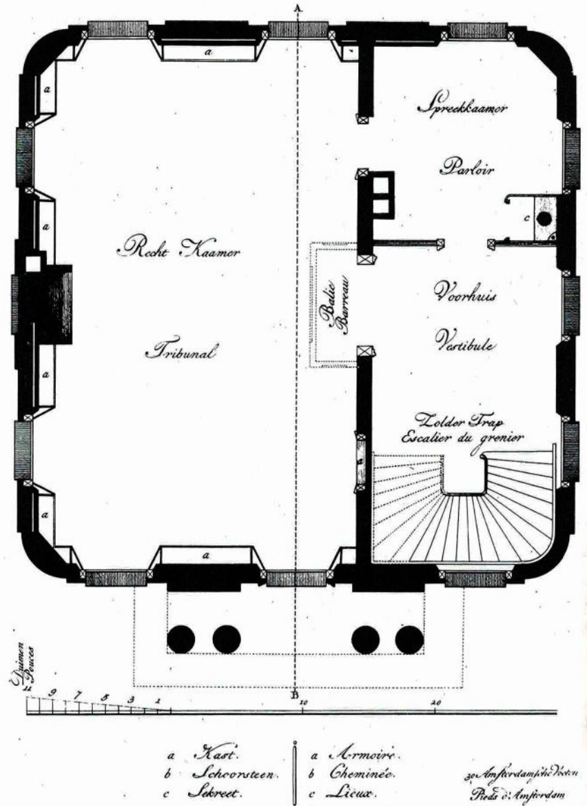
PLATTEGROND VAN DE TWEDE VERDIEPING | PLAN DU SECOND ETAGE
